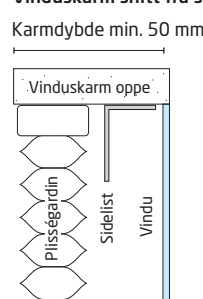
Vinduskarm snitt fra siden
